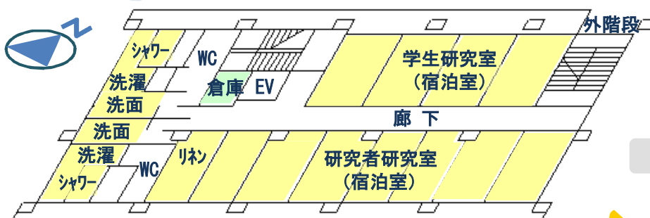
3 F 平面図
